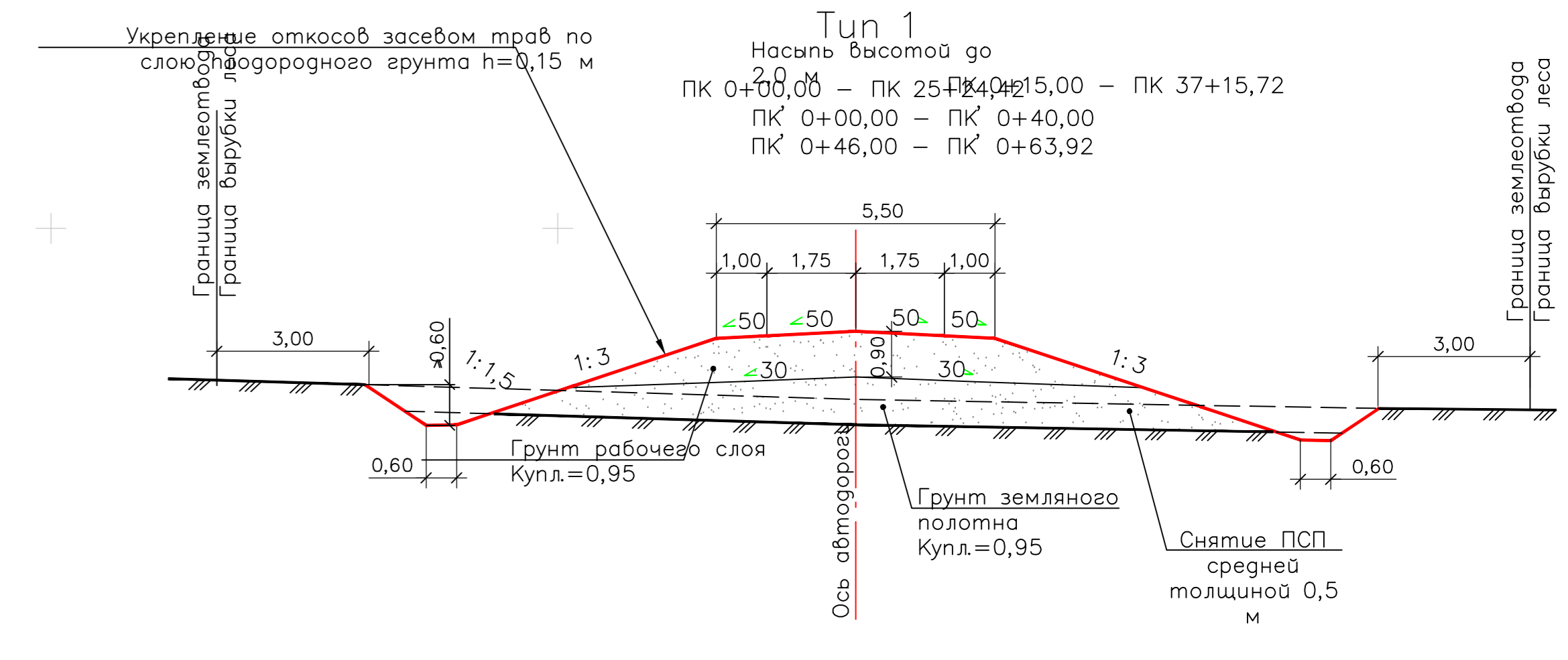
Конструктивные поперечные профили земляного полотна (1:100)
